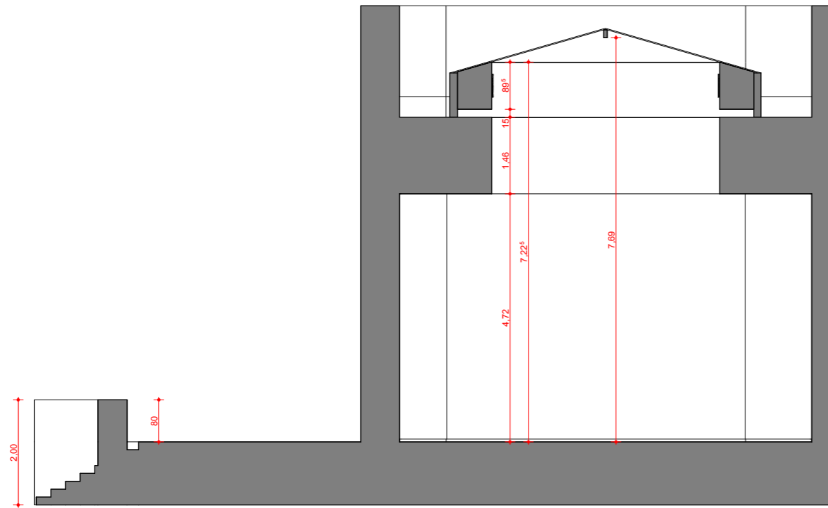
SECTIUNEA E-E
