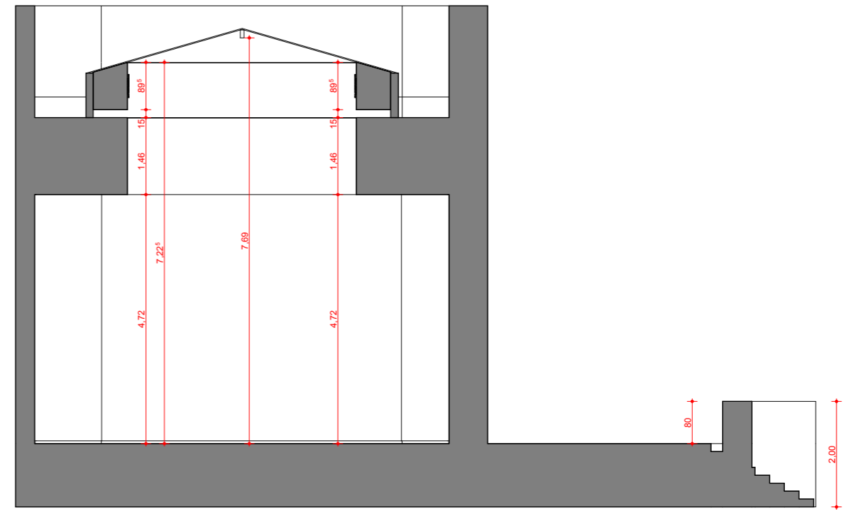
SECTIUNEA F-F
