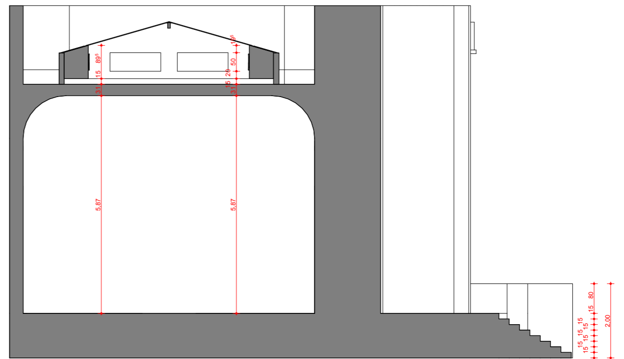
SECTIUNEA C-C
