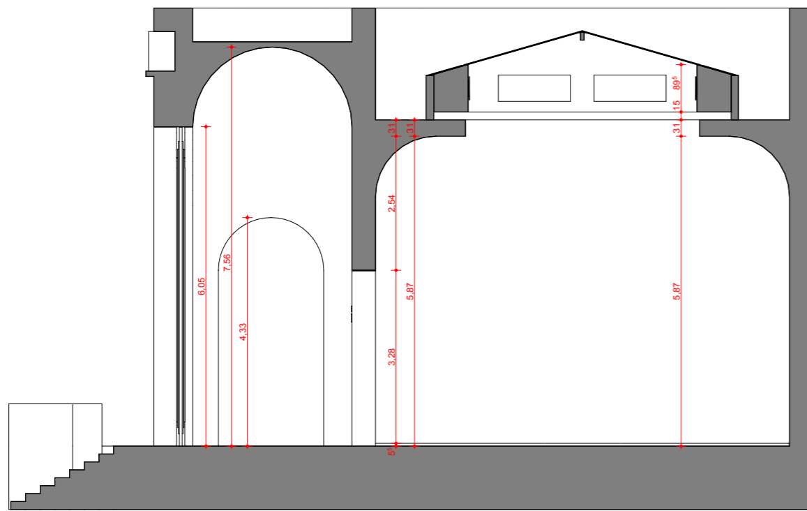
SECTIUNEA B-B
