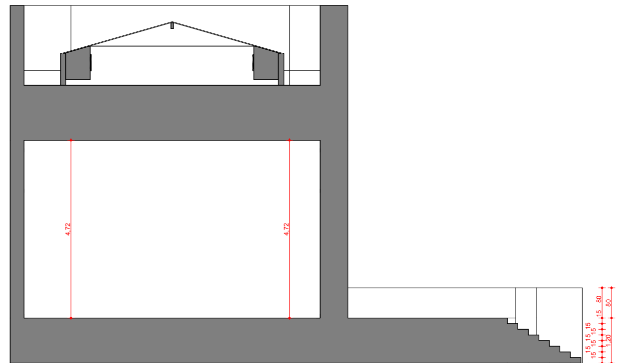
SECTIUNEA H-H
