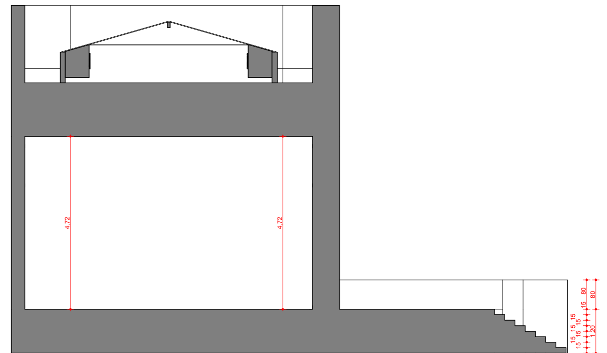
SECTIUNEA H-H
