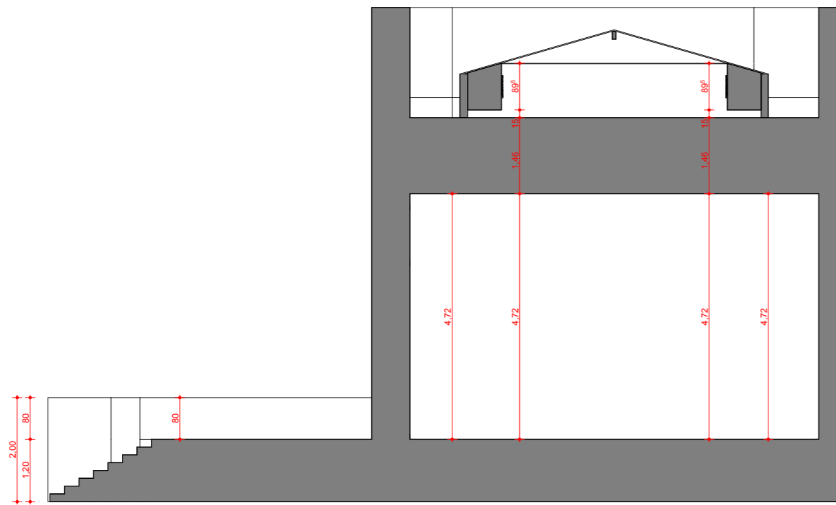
SECTIUNEA I-I
